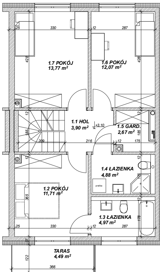
RZUT PIĘTRA
