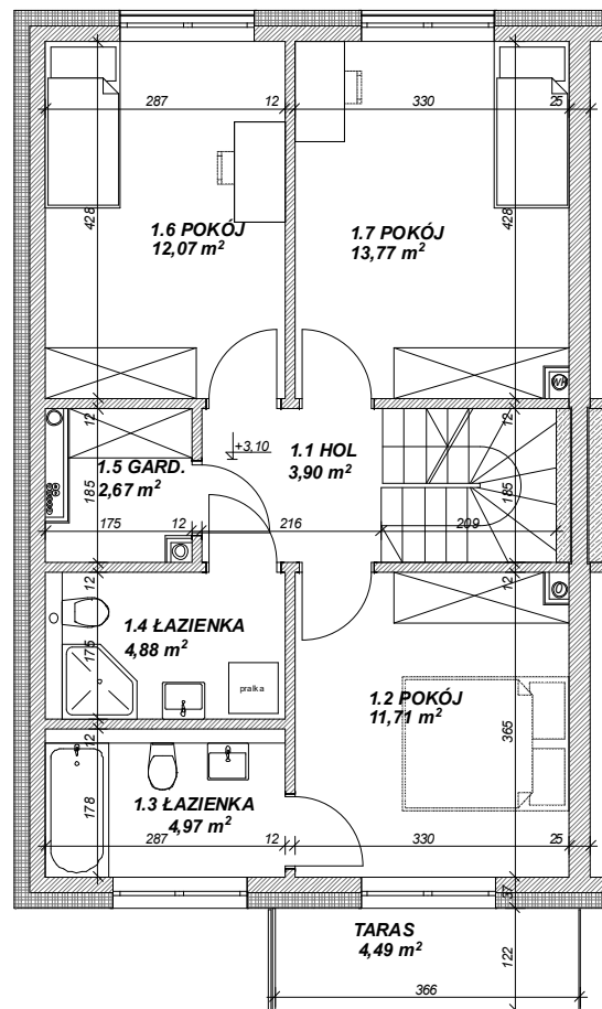
RZUT PIĘTRA
