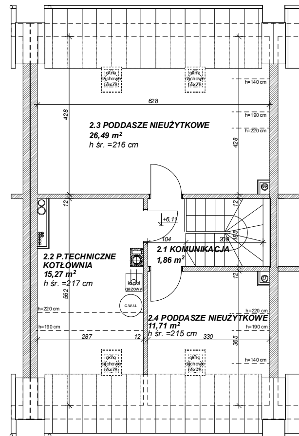
RZUT PODDASZA
